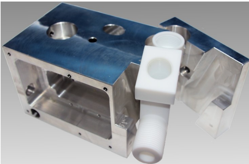
Aluminium Frästeil für die Umweltmesstechnik mit PTFE-Einsatzstück—messblock für Messung von pH-Wert und elektrischer Leitfähigkeit.
