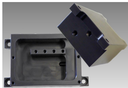
POM Frästeil für Biotechnologie und Dosier-Technik.
